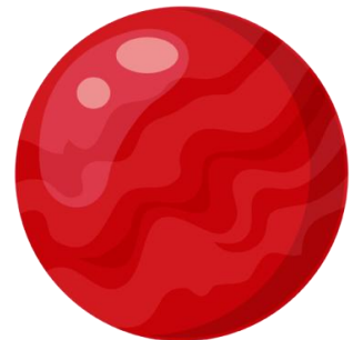
Mars
